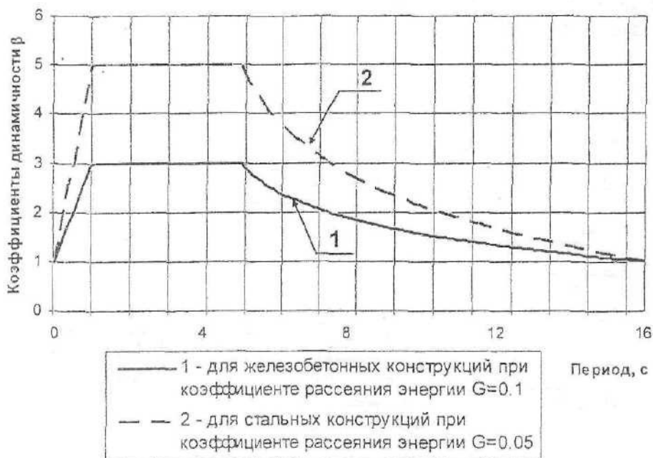
Графики коэффициентов динамичности \beta
