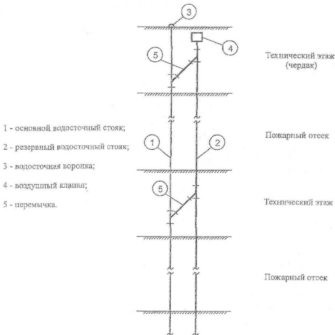
Рис. 8.1. Схема водостока с устройством резервного стояка
